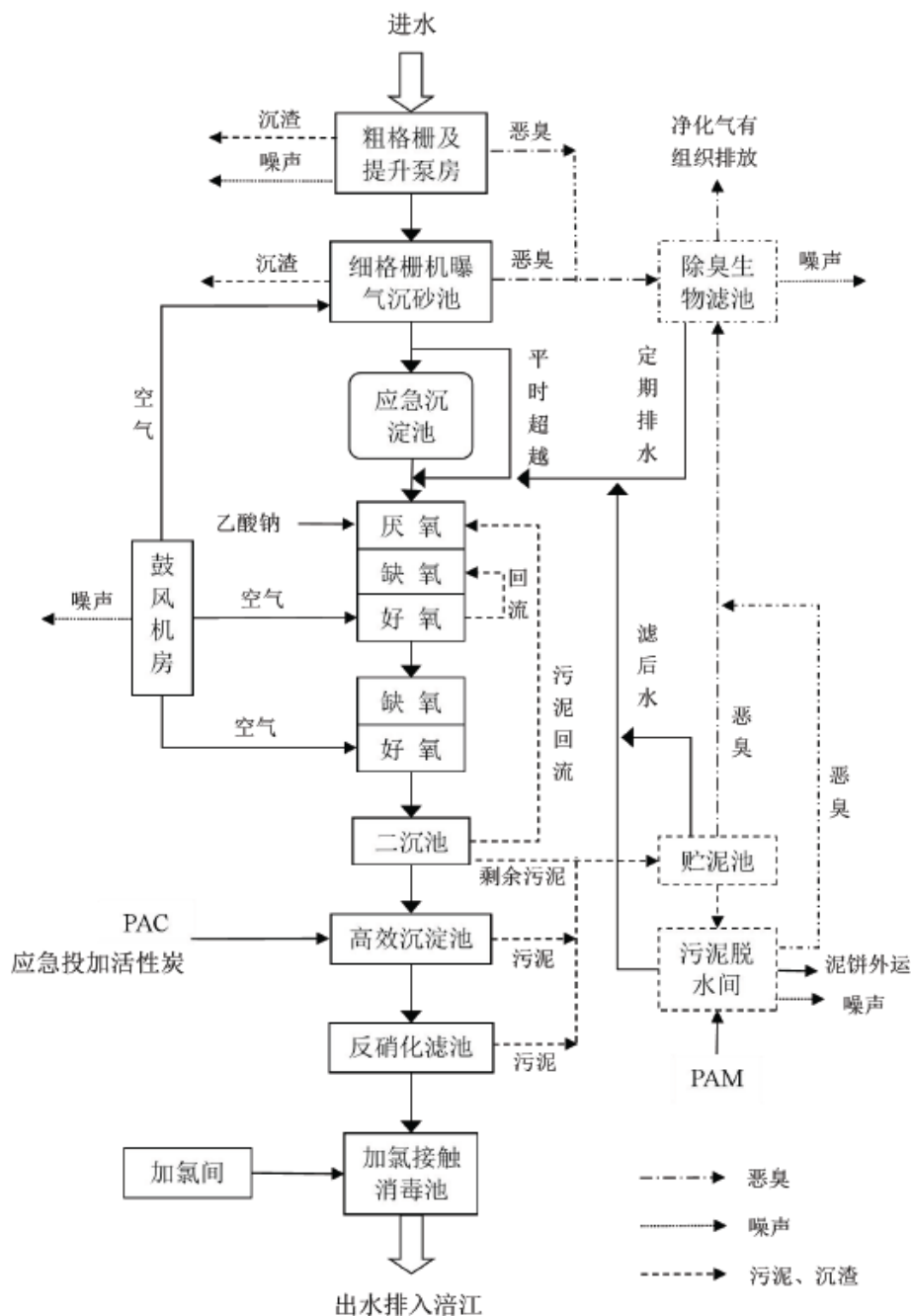
图 3.4-3 城南第二污水处理厂工艺流程图
